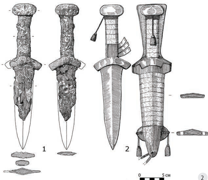
Рис. 1. Кинжал из кургана №25 могильника Ханкаринский дол. 2 – реконструкция кинжала в ножнах (по: Дашковский, 2020в; 2021а)
