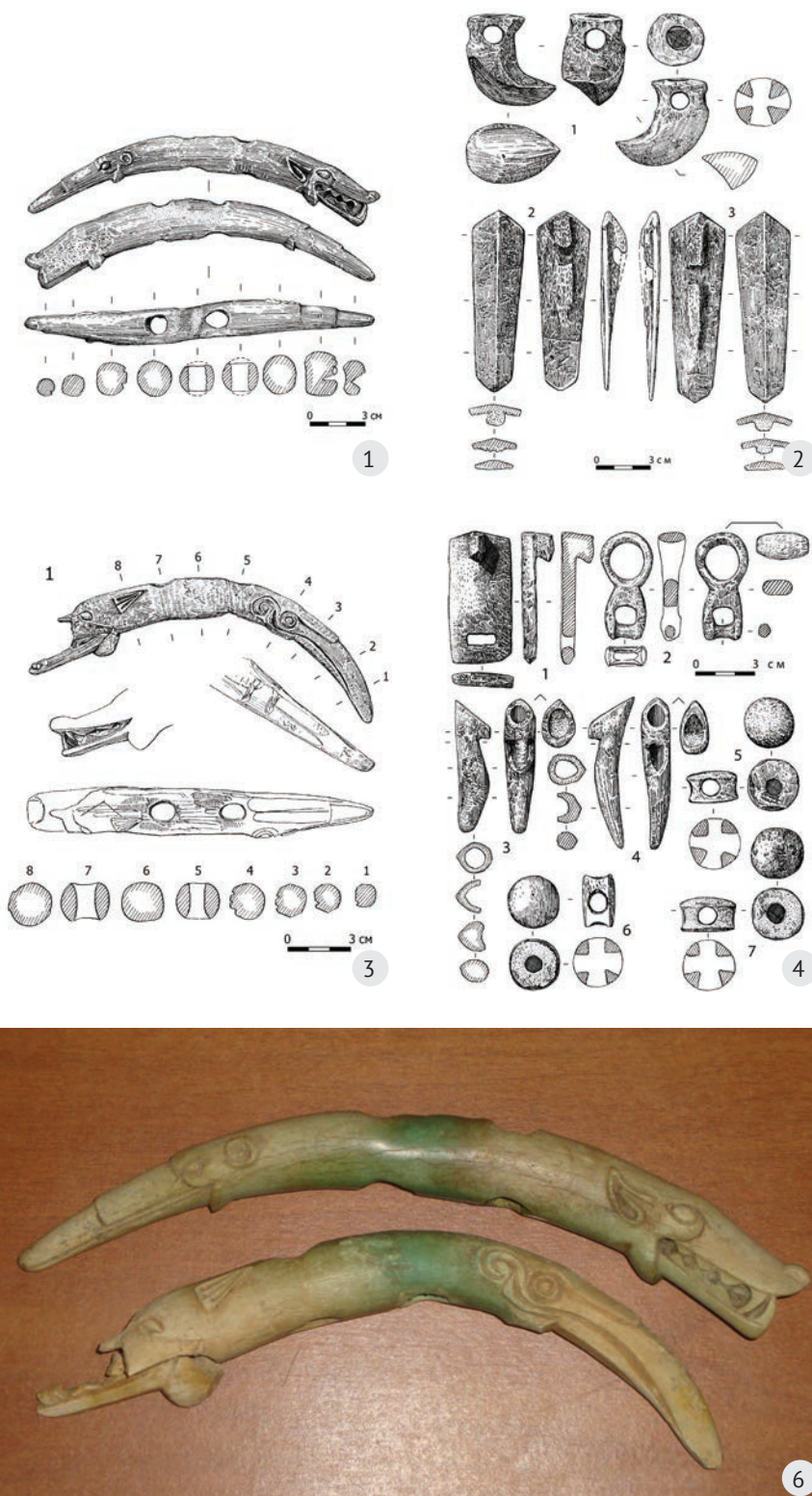
Рис. 3. Роговой псаий из кургана №25 могильника Ханкаринский дол (по: Дашковский, 2020в)
