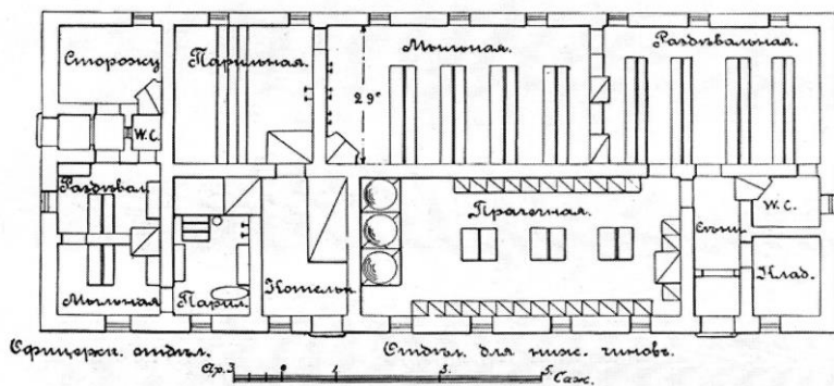
Рис. 20. План типовой войсковой бани
