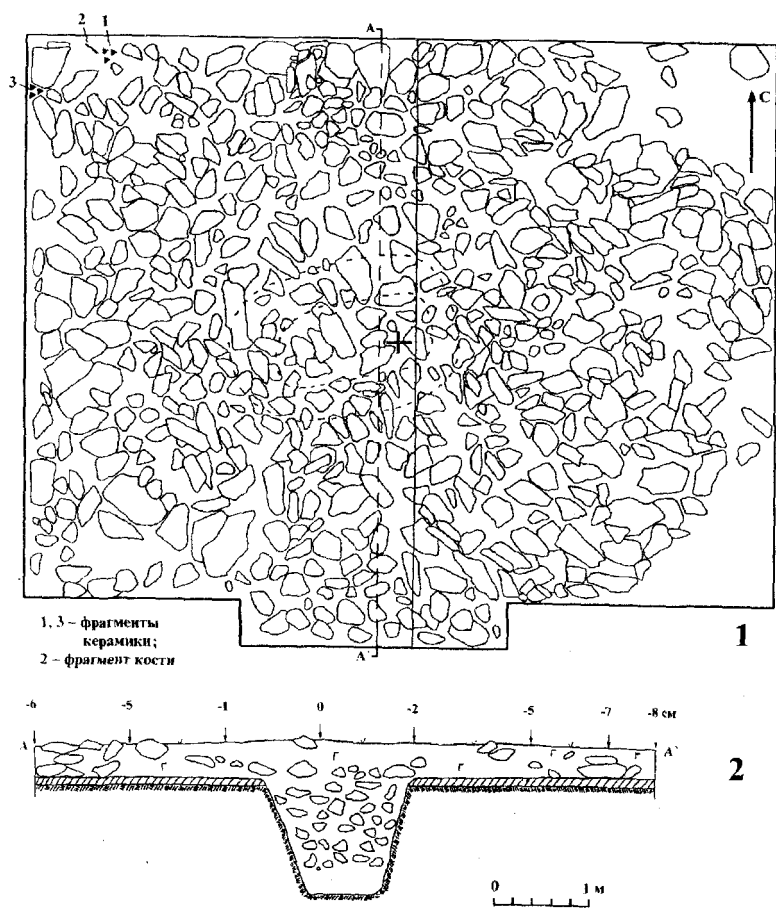
Рис. 77. Курган №33. План насыпи (1) и разрез сооружения (2)
