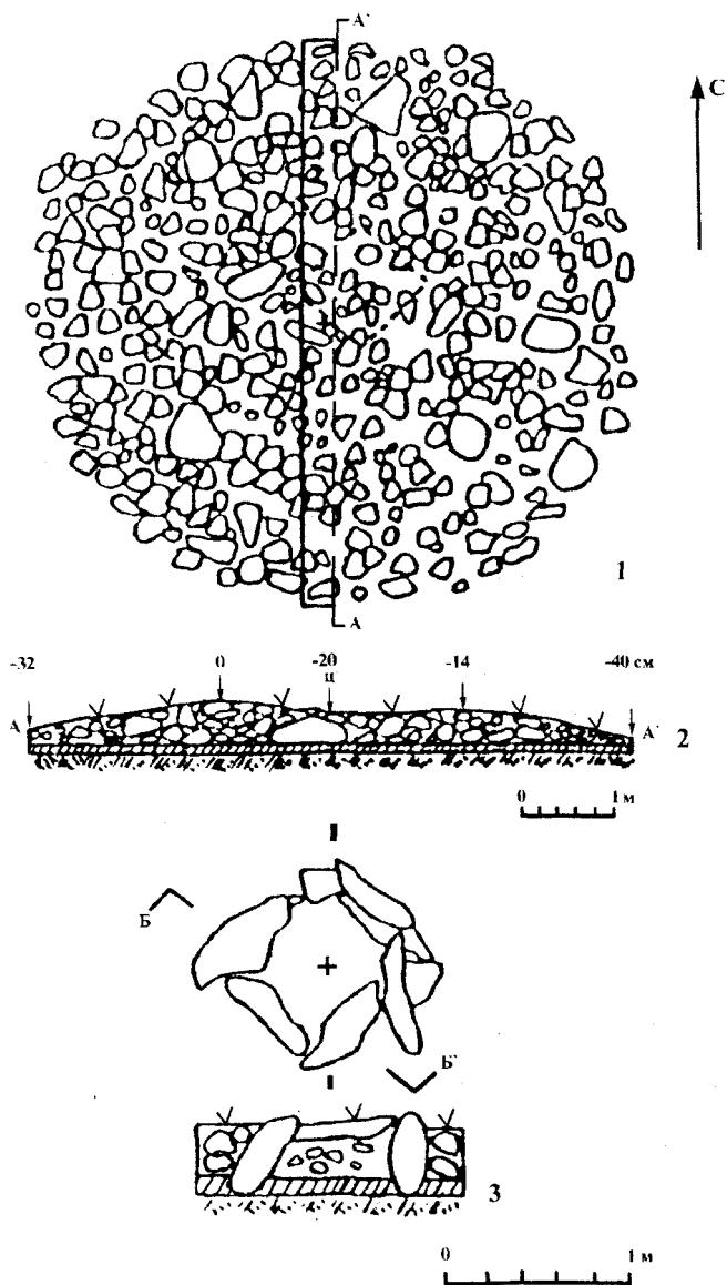
Рис. 3. Курган №1. План (1) и разрез насыпи (2). Каменный ящик (3)
