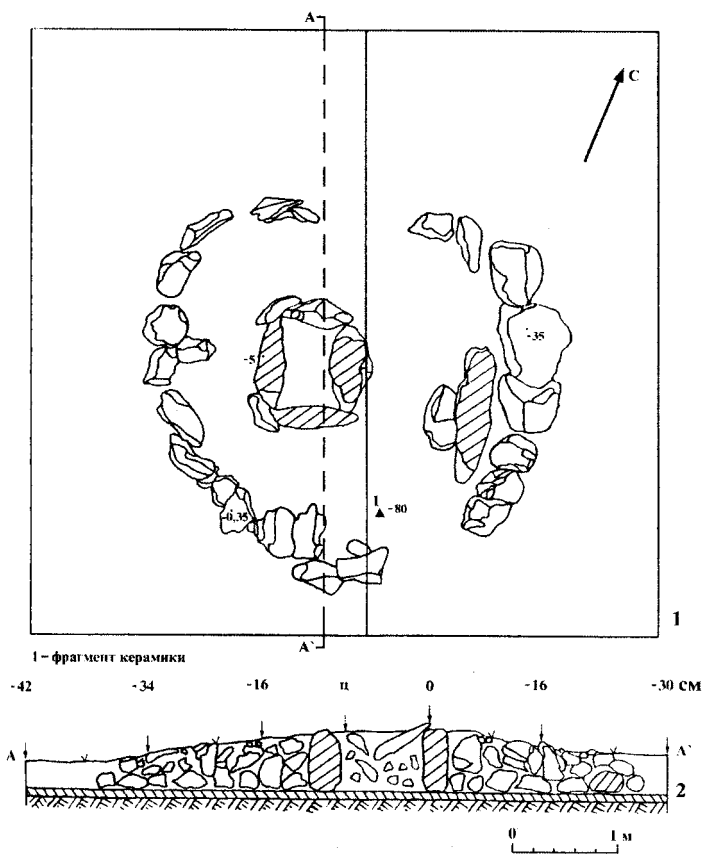
Рис. 16. Курган №16. План кольца с каменным ящиком (1). Разрез объекта (2)
