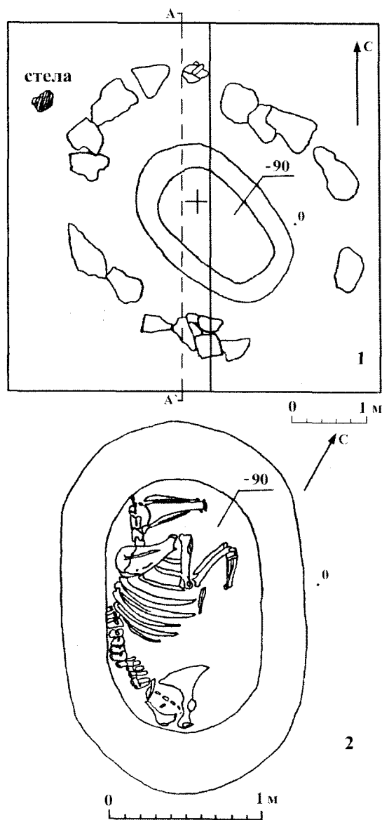
Рис. 53. Выкладка №45. План каменного кольца и ямы (1). Захоронение лошади (2)
