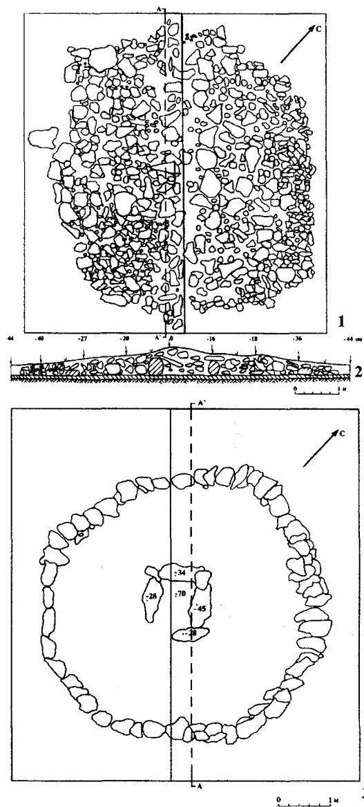
Рис. 24. Курган №19. План (1) и разрез насыпи (2). План кольца с каменным ящиком (3)
