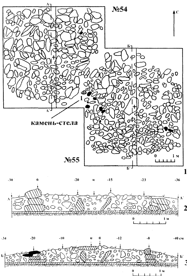
Рис. 63. Курганы №54 и 55. Планы насыпей (1) и разрезов (2, 3)
