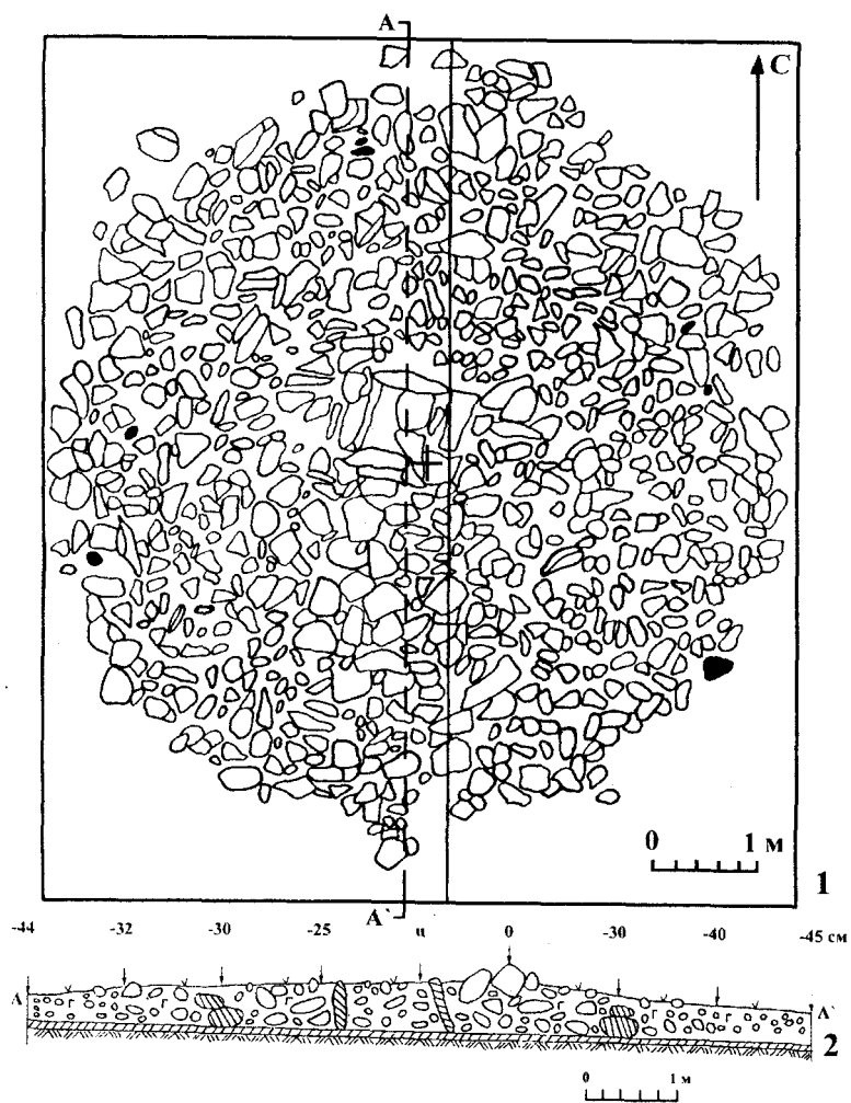
Рис. 67. Кургan №57. План насыпи (1) и ее разреза (2)
