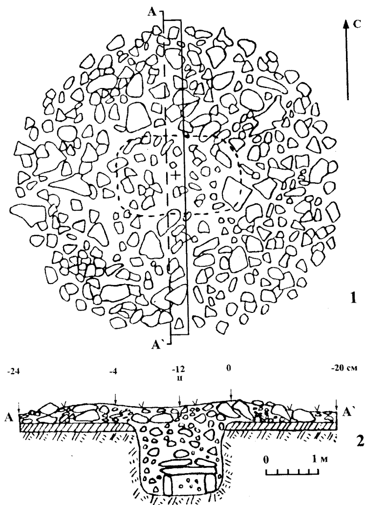
Рис. 89. Кургan №3. План насыпи (1). Разрез сооружения (2)
