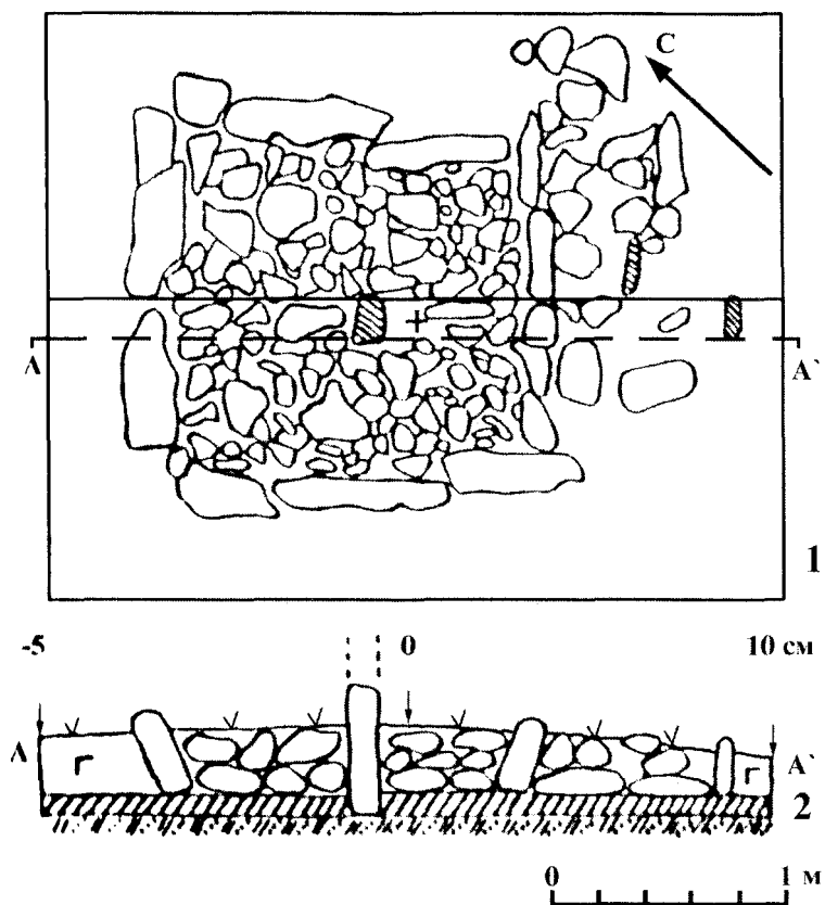
Рис. 100. Оградка №8. План (1) и разрез объекта (2)
