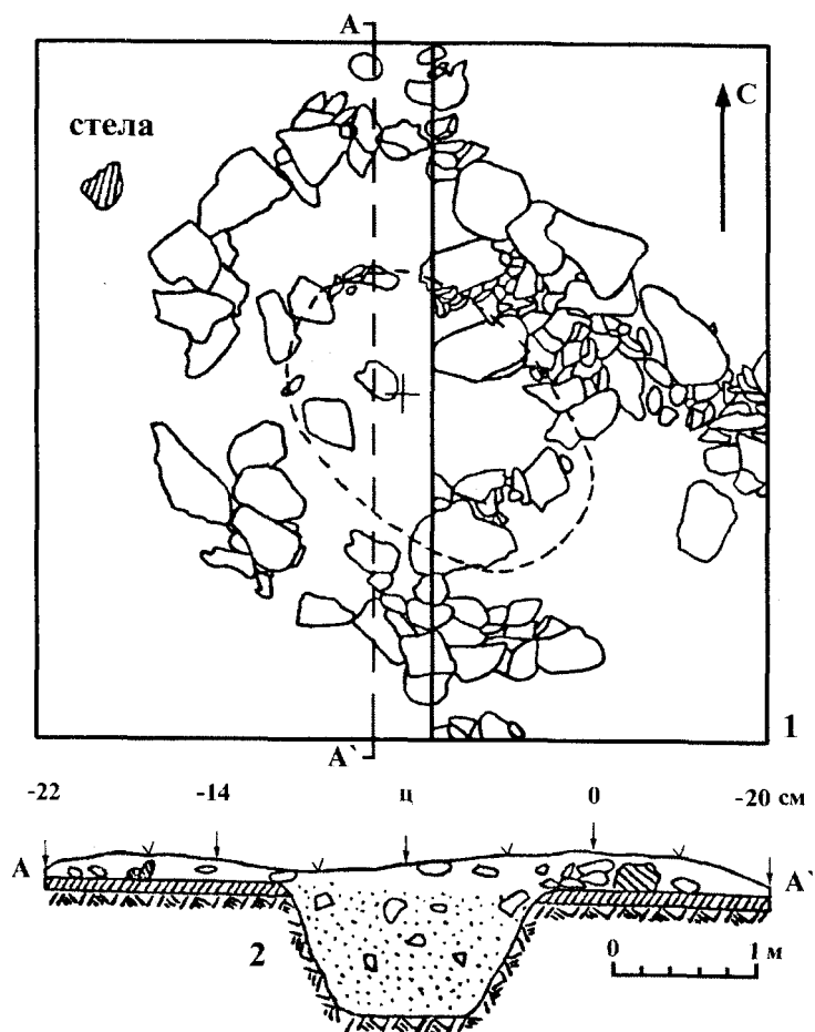
Рис. 52. Выкладка №45. План (1) и разрез объекта (2)
