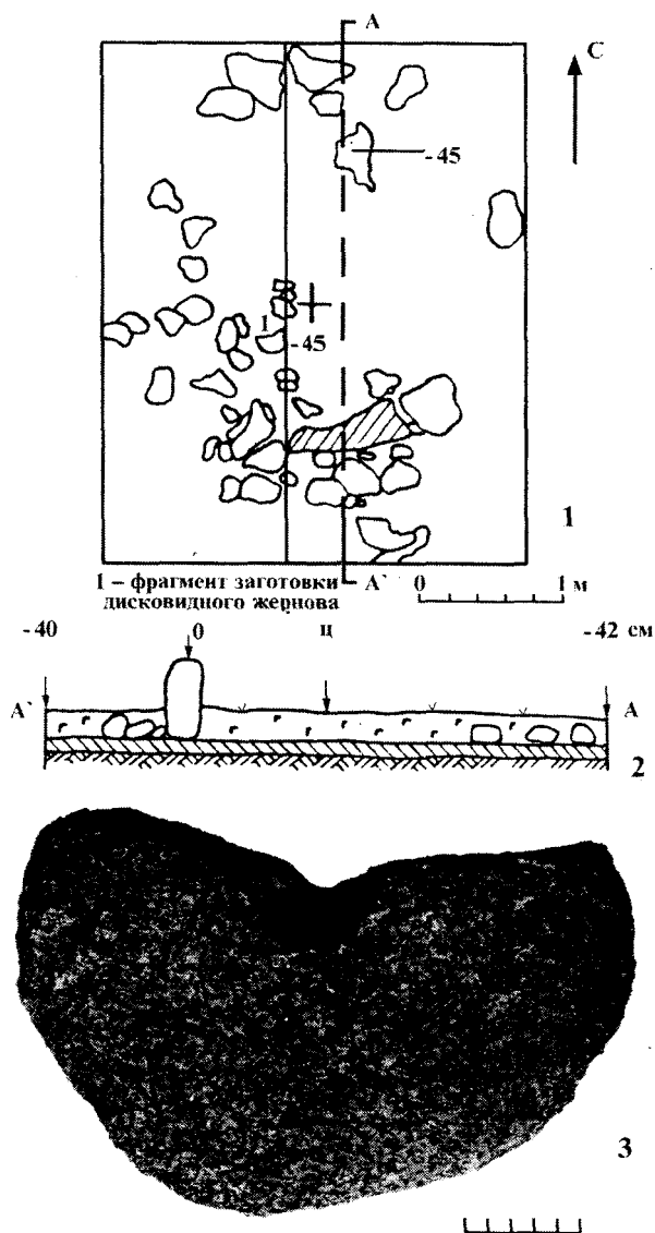
Рис. 34. Выкладка №25. План (1) и разрез (2) объекта. Заготовка дисковидного жернова (3) из серого гранита (фото)
