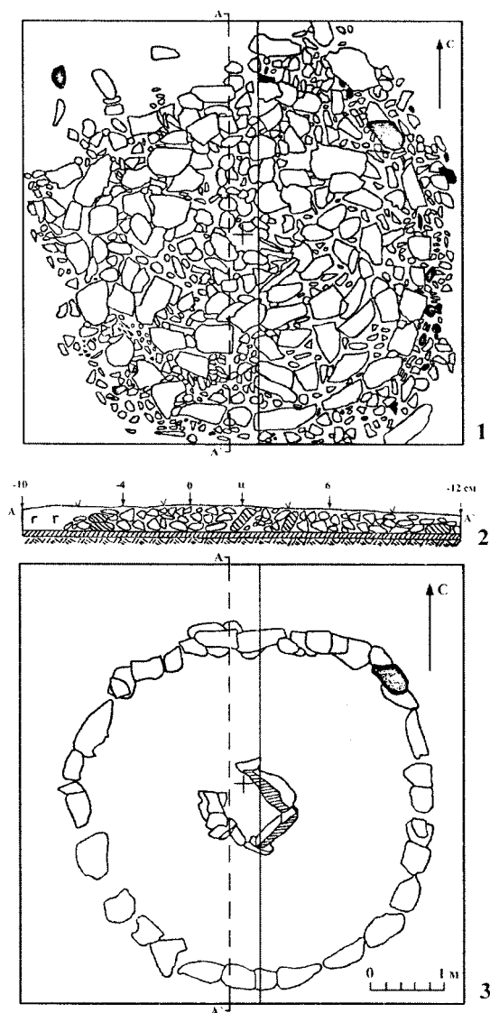
Рис. 58. Кургan №47. Планы насыпи (1), разреза (2) и каменного кольца с ящиком (3)
