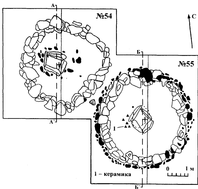
Рис. 64. Курганы №54 и 55. Планы колец с ящиками
