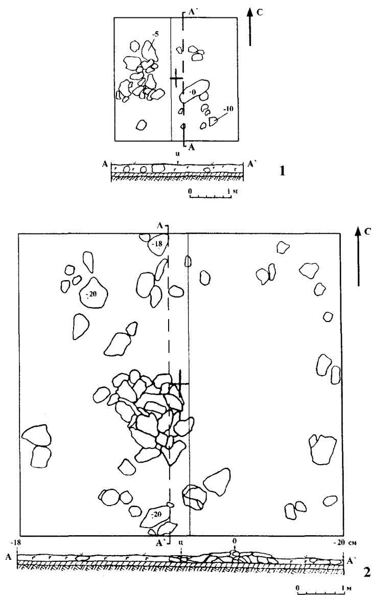
Рис. 43. Планы и разрезы: 1 – выкладка №35; 2 – выкладка №36
