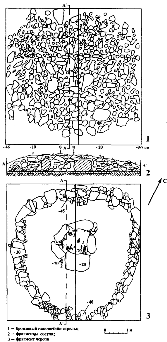
Рис. 28. Курган №21. Планы насыпи (1). Разрез сооружения (2). Каменное кольцо с ящиком (3)
