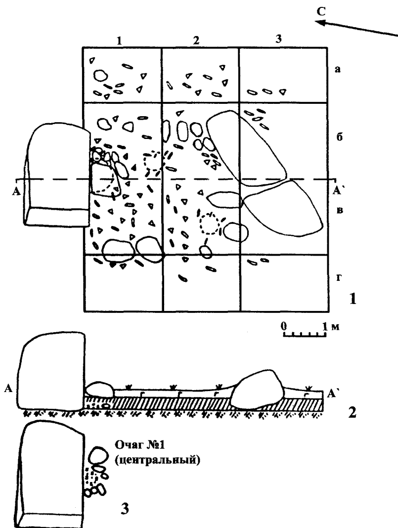
Рис. 86. План раскопа на святилище у камня (1) и его разрез (2). Очаг №1 (3)
