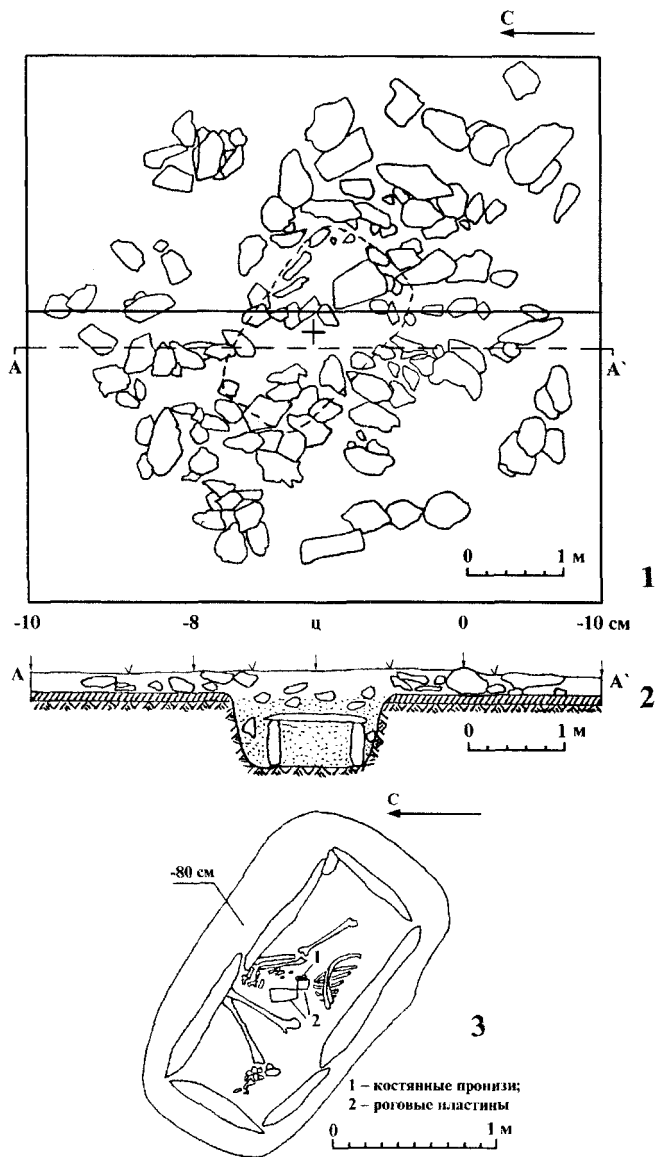
Рис. 98. Курган №42. 1, 2 – план насыпи и разрез сооружения; 3 – план погребения
