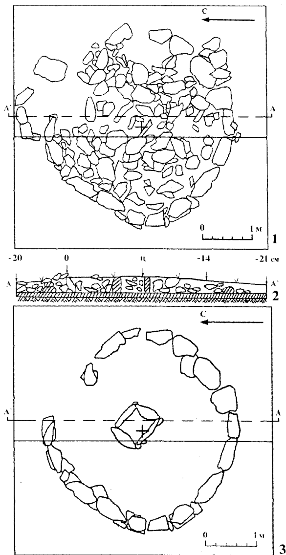
Рис. 51. Кургan №44. Насыпь (1) и ее разрез (2). Кольцо с каменным ящиком (3). Планы
