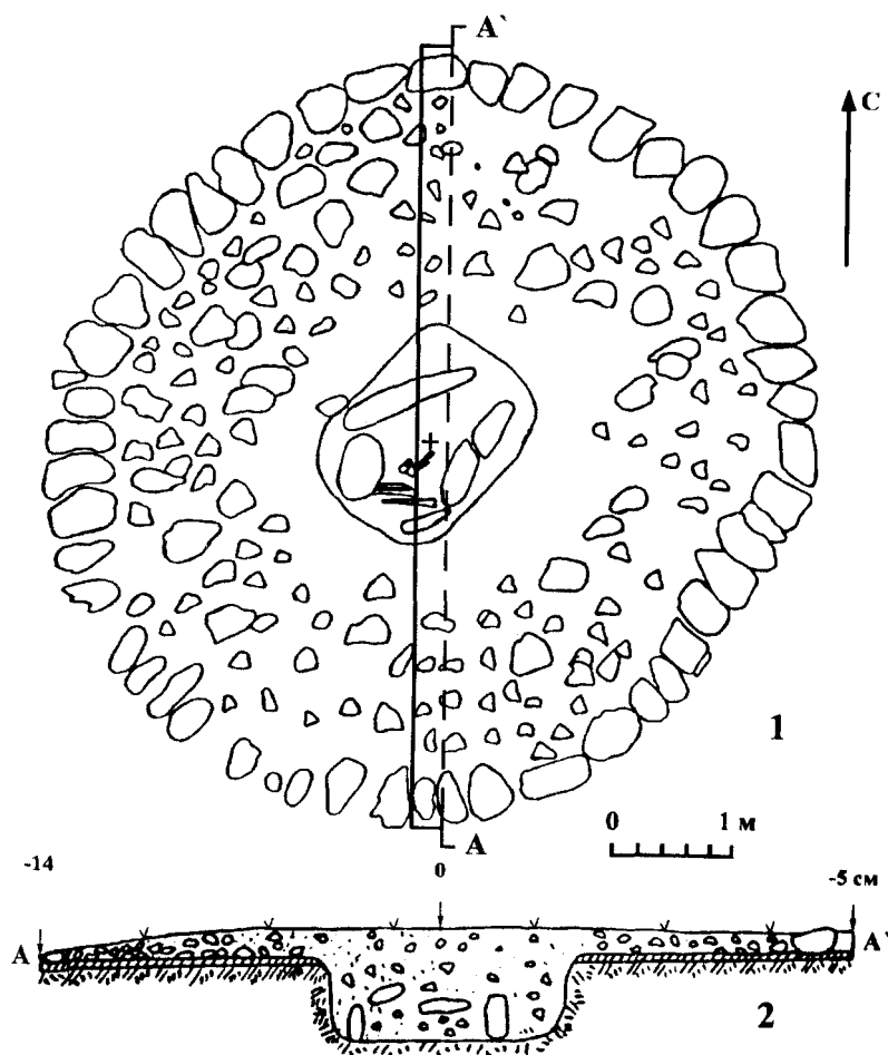
Рис. 88. Кургan №2. План насыпи (1). Разрез сооружения (2)
