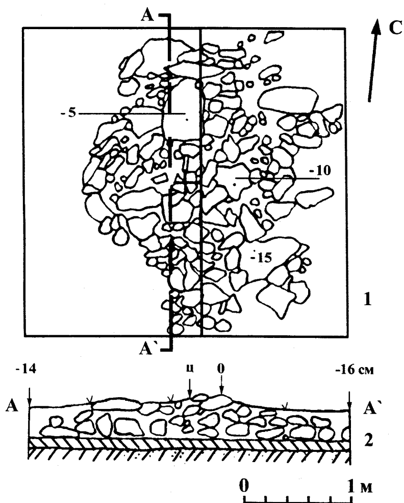
Рис. 33. Выкладка №24. План (1) и разрез объекта (2)
