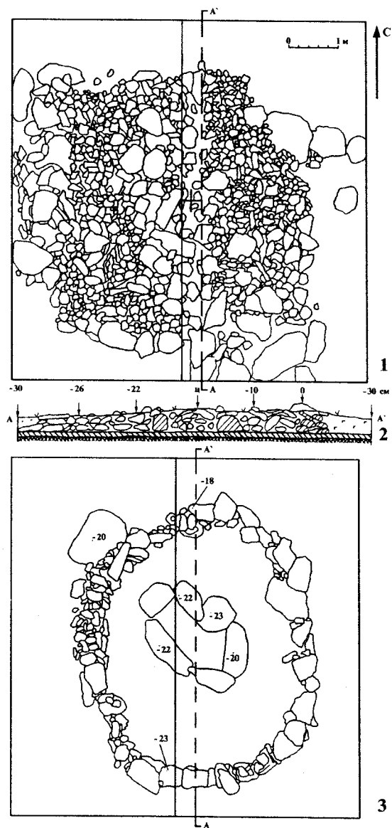
Рис. 35. Курган №28. Насыпь (1), разрез сооружения (2) и кольцо с ящиком (3). Планы
