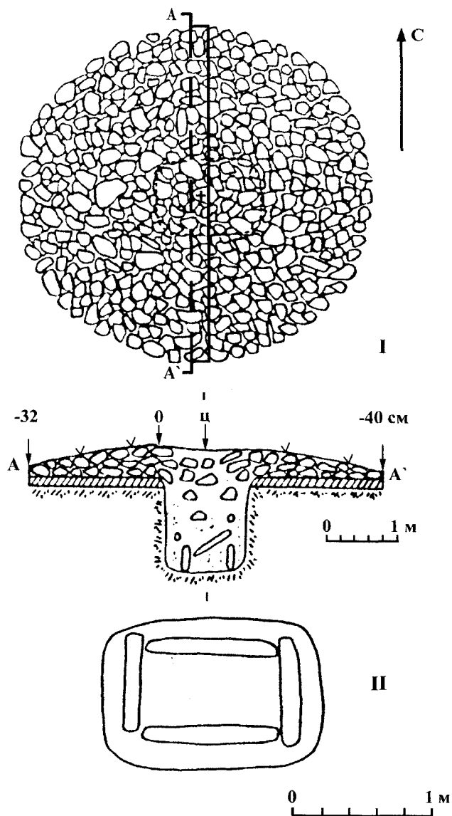
Рис. 94. Кургan №10. План насыпи и разрез сооружения (I). Каменный ящик (II)
