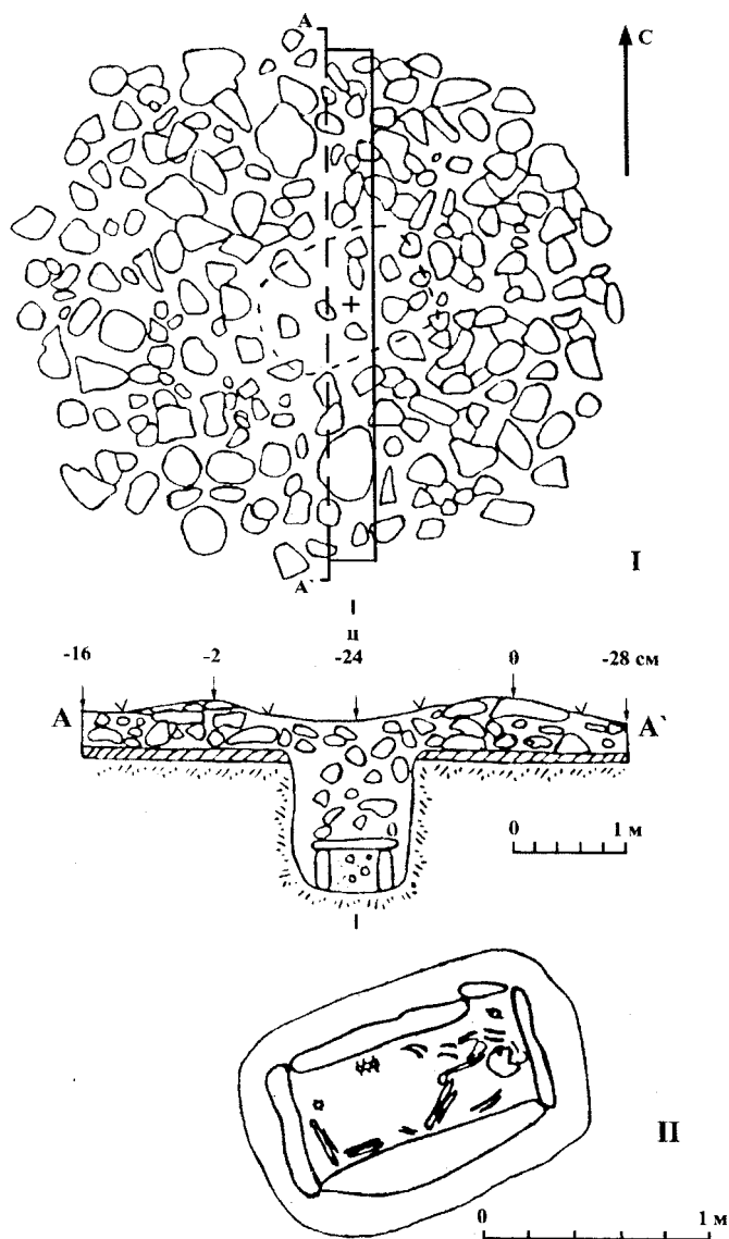
Рис. 93. Курган №5. I – план насыпи и разрез сооружения; II – план погребения
