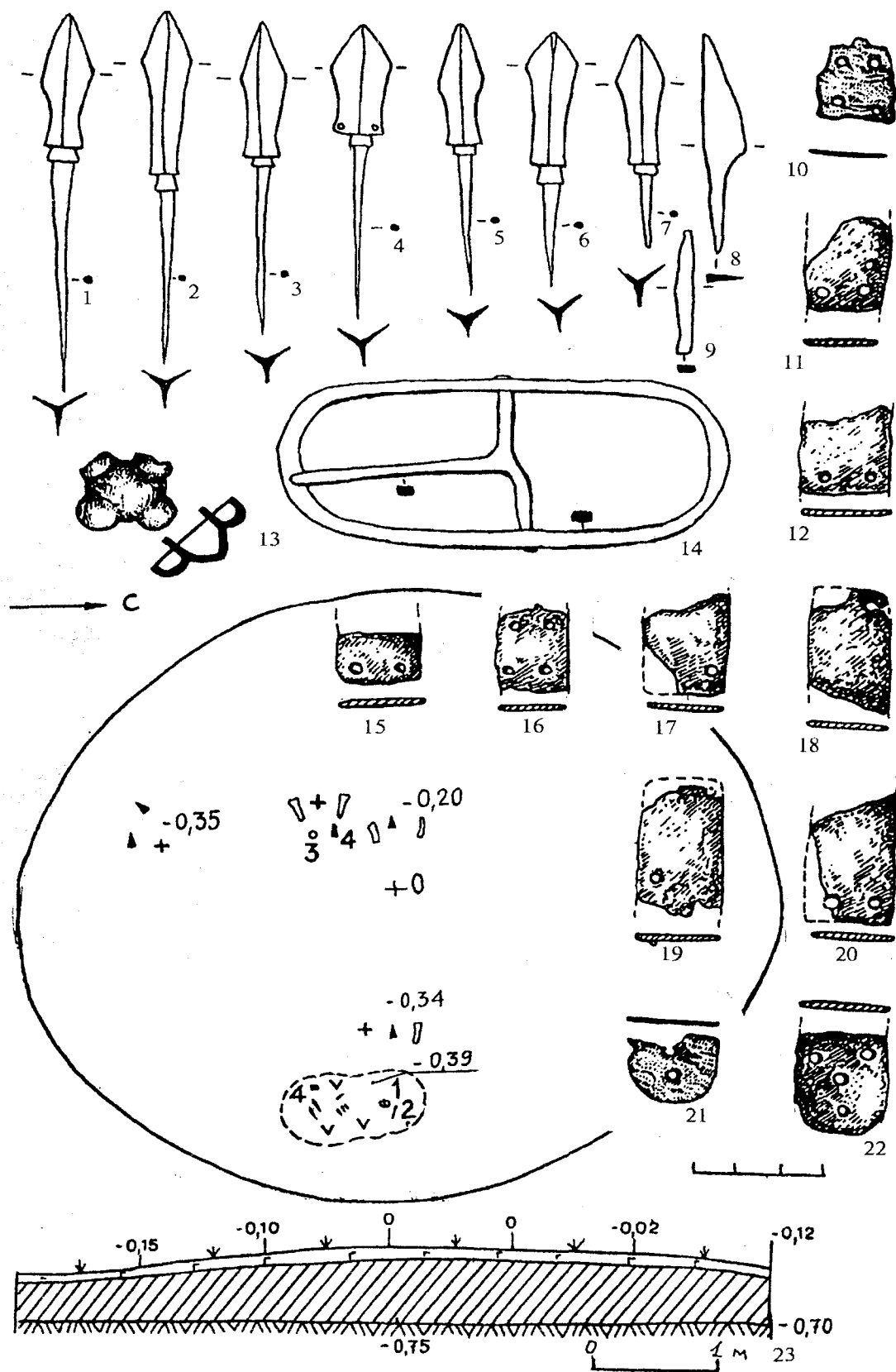
Рис. 12. Гилево-III, курган 10: 1-7 – наконечники стрел; 8 – нож; 9 – шило, проколка; 10-12, 15-22 – фрагменты панцирных пластин; 13 – бляшка; 14 – подпружная пряжка. 13 – медь, остальное – железо. 23 – план и разрез кургана (1 – подпружная пряжка; 2 – семь железных трехлопастных наконечников стрел; 3 – медная бляшка; 4 – панцирные пластины)
