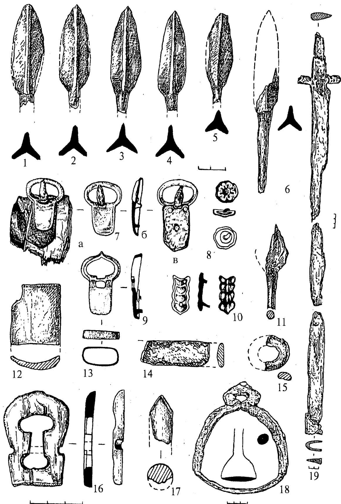
Рис. 25. Гилево-V, курган 6: 1-6, 11 – наконечники стрел; 7 – пряжка с остатками ремня и бересты от колчана; 8 – бляшка; 9 – пряжка от подвески палаша; 10 – наконечник ремня; 12 – накладка; 13 – обойма; 14 – нож; 15 – уздечное кольцо; 16 – пряжка; 17 – обломок костяного предмета; 18 – стремя; 19 – палаш с наконечником ножен. 1-6, 11, 14, 15, 18, 19 – железо; 7-10, 13 – медно-серебряный сплав; 12, 16, 17 – кость. 8-10, 13, 15, 18 – по 2 экз.
