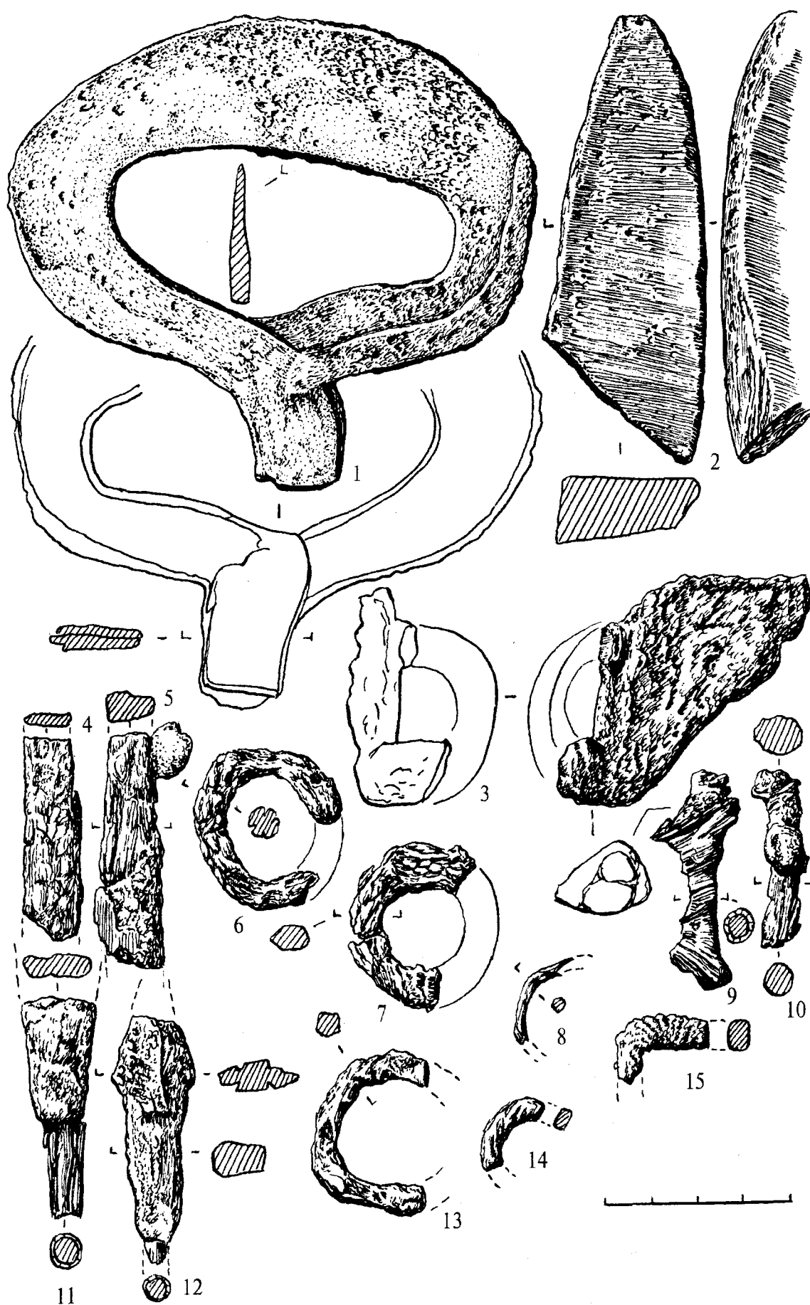
Рис. 12. Ильинка: 1 – кресало из ямы в траншее 11; 2 – тогильный камень из могилы 5; остальное – сборы на выдувах. 1, 3–8, 13–15 – железо; 2 – камень; 9–12 – железо, дерево
