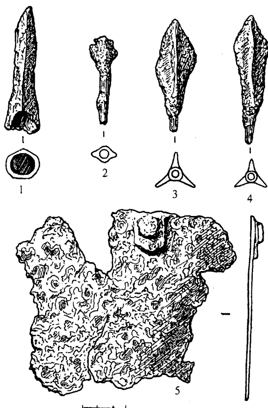
Рис. 33. Корболиха-II, курган 7: 1 – наконечник копья; 2–4 – наконечники стрел; 5 – венчик котла (железо)
