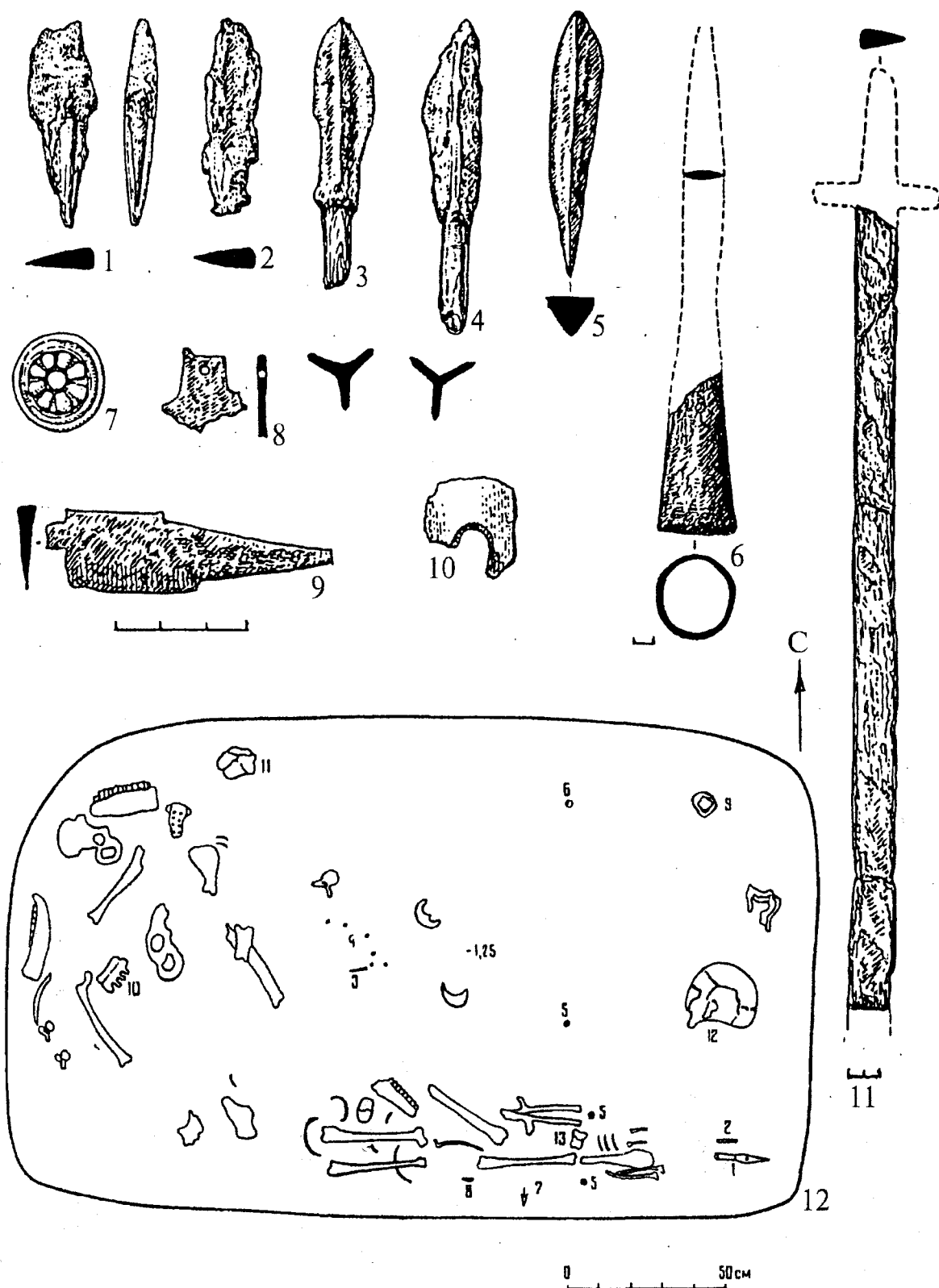
Рис. 18. Гилево-IV, курган 1: 1, 2, 9 – обломки ножей; 3–5 – наконечники стрел; 6 – наконечник копья; 7 – бронзовая бляшка; 8 – фрагмент панцирной пластины; 10 – обломок костяного предмета; 11 – фрагменты клинка палаша; 12 – план погребения (1 – наконечник копья; 2 – обломок костяного предмета; 3 – обломки ножа; 4 – фрагменты железных предметов; 5 – панцирные пластины; 6 – бляшка; 7 – наконечники стрел; 8 – черешки от наконечников стрел; 9 – копыта лошади; 10 – крестец лошади; 11, 12 – черепа взрослых; 13 – череп ребенка)
