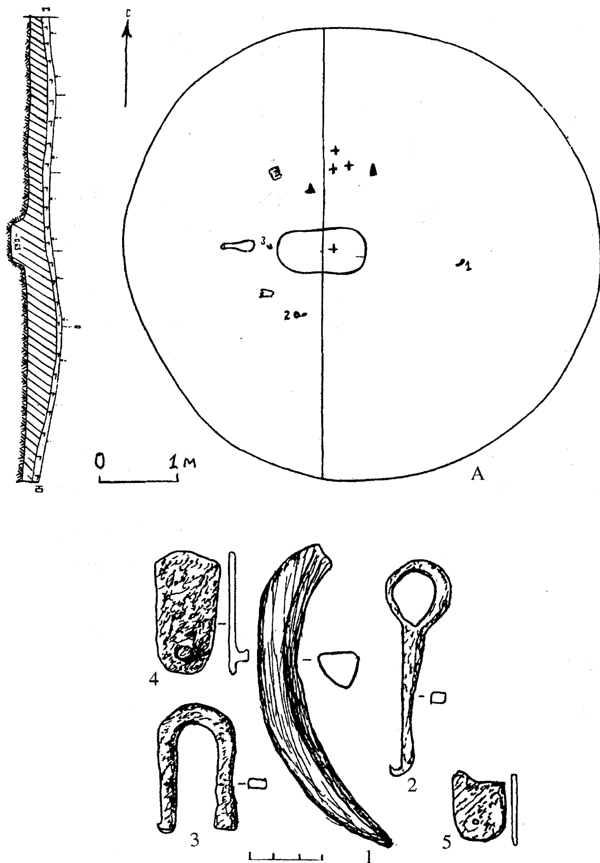
Рис. 8. Гилево-III. А, 1-3 – курган 4; 4 – курган 2; 5 – курган 14. 1 – клык кабана; 2-5 – железо
