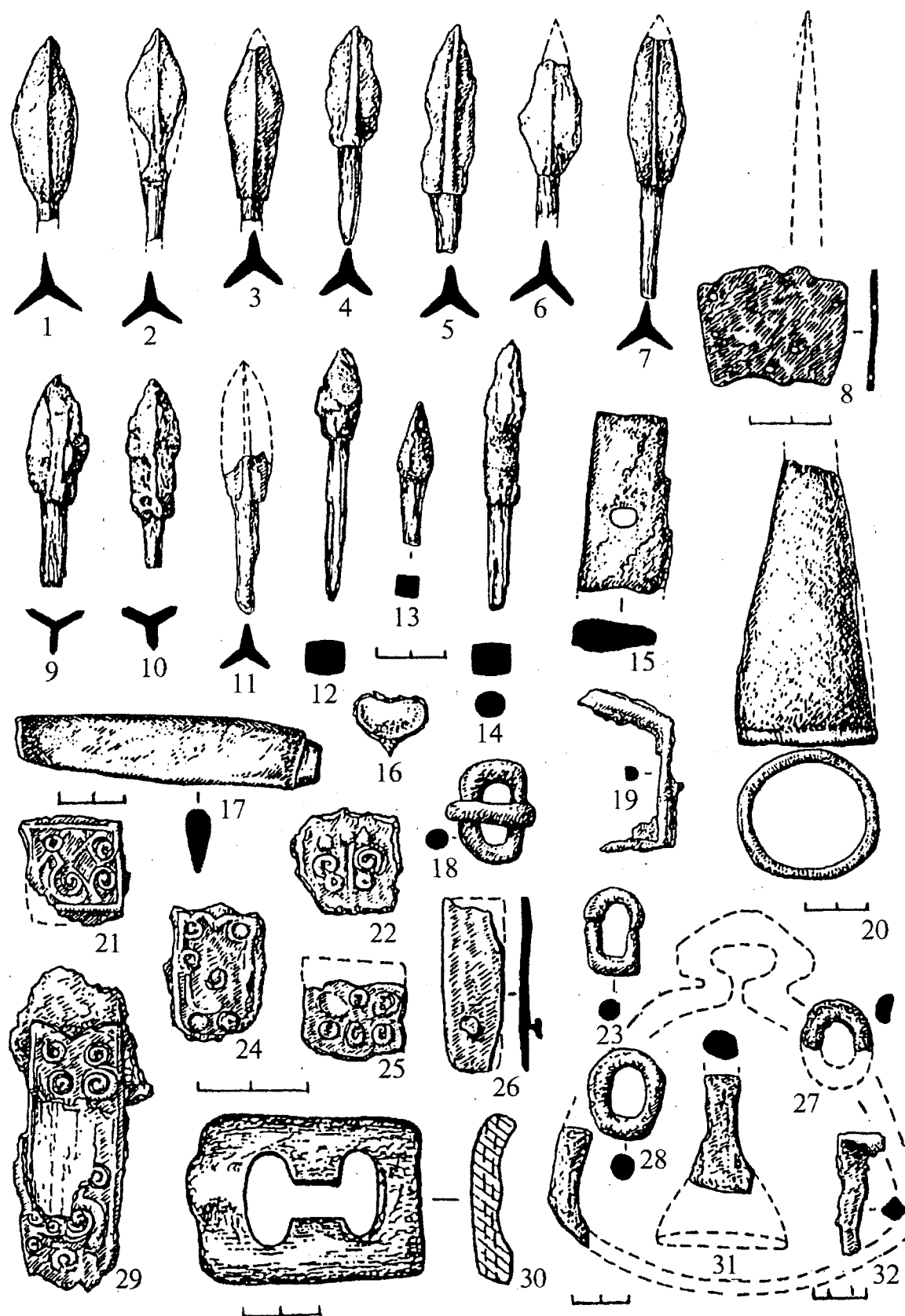
Рис. 23. Гилево-V, курган 5: 1-7, 9-14 – наконечники стрел; 8 – панцирная пластина; 15 – фрагмент рукояти палаша; 16 – бляшка; 17 – нож с остатками ножен; 18, 19, 23, 30 – пряжки (19, 30 – подпружные); 20 – втулка от наконечника копья; 21, 22, 24-26, 29 – бляхи и наконечники ремней; 27, 28 – уздечные кольца; 31 – фрагмент стремени; 32 – гвоздь. 1-15, 18-20, 23, 26-28, 31, 32 – железо; 16 – медь; 17 – железо с остатками дерева от ножен; 21, 22, 24, 25, 29 – железо с золотой инкрустацией; 30 – кость
