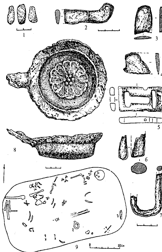
Рис. 27. Гилево-V, курган 7: 1 – подвески из резцов марала; 2 – обломки ножа; 3, 4 – фрагменты железных предметов; 5 – пряжка; 6 – обломок заполированной рукояти (?); 7 – обломок крючко-видного предмета; 8 – жаровня. 2-4, 7 – железо; 5, 6 – рог, кость; 8 – чугун; 9 – план погребения (1 – подвески из резцов марала; 2 – жаровня; 3 – пряжка; 5 – развал котла; 6 – крючок; 7 – обломки железных предметов)
