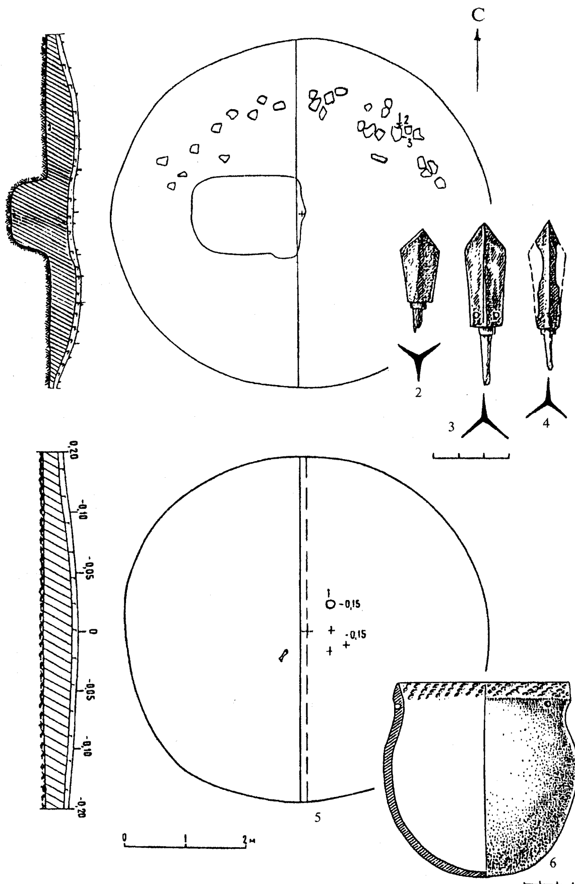
Рис. 13. Гилево-III: 1-4 – курган 12; 5, 6 – курган 22. 2-4 – железо; 6 – глина
