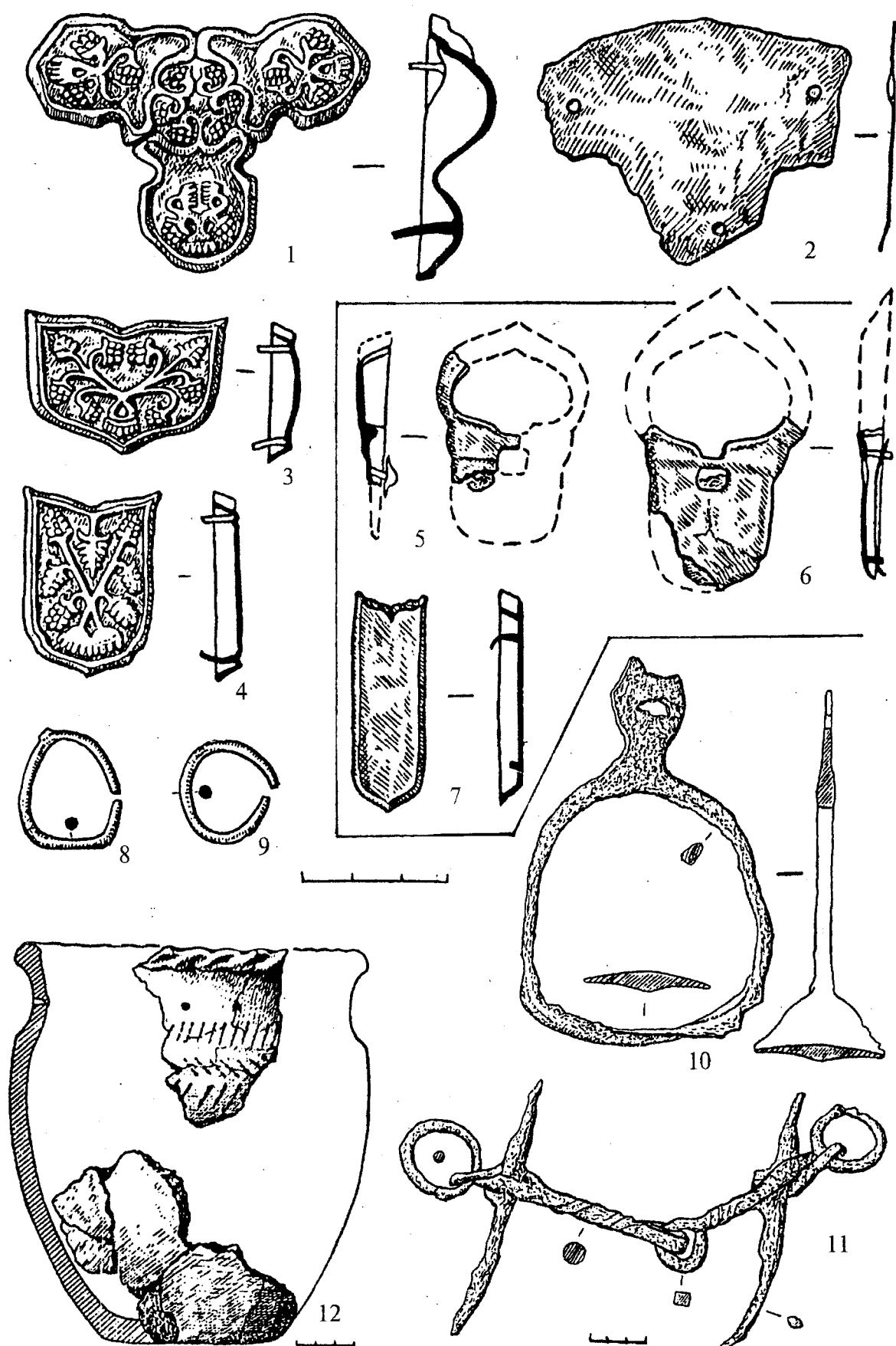
Рис. 37. Корболиха-VIII, курган 5: 1–4, 8–12 – погребение 2, с кремацией; 5–7 – центральное погребение 1 (кенотаф – ?). 1, 3, 4 – бронза с позолотой; 2, 5–7 – бронза; 8, 9 – золото; 10, 11 – железо; 12 – глина (1, 7 – по 2 экз.; 3–4 экз.)
