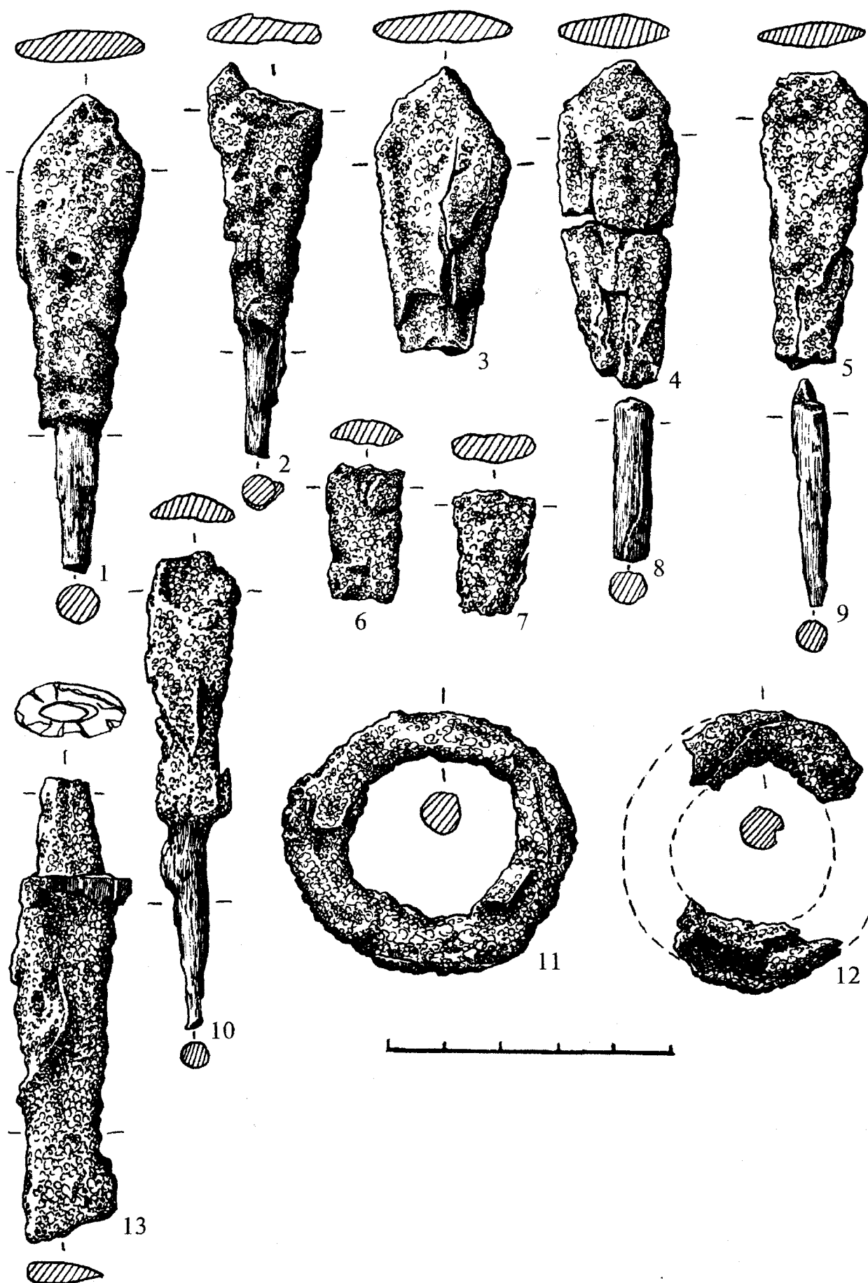
Рис. 1. Остатки железных наконечников стрел (1–10), колец (11–12) и ножа (13) из могилы 3 памятника Сухие Гривы
