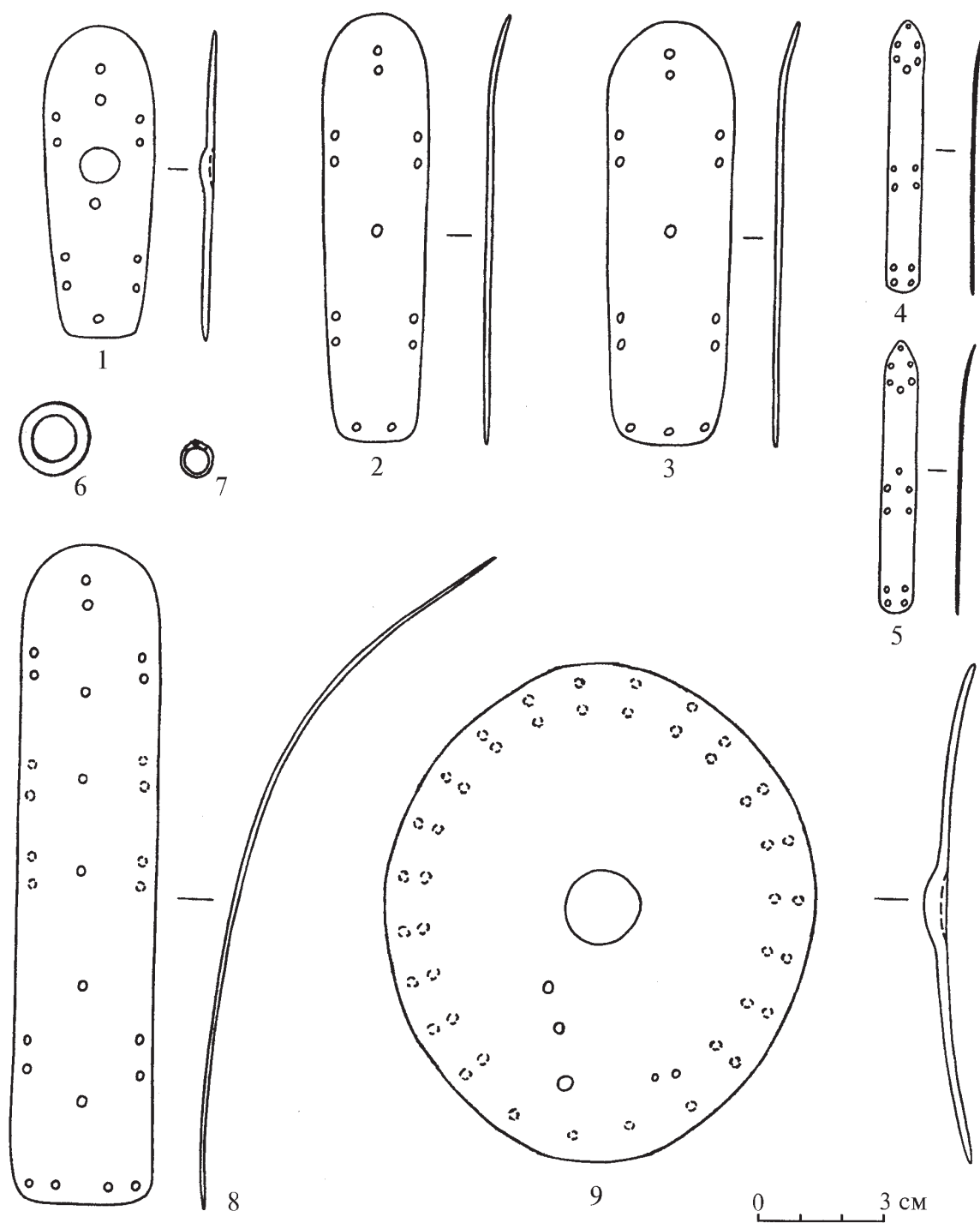
Рис. 10. Реконструированные панцирные пластины и наверхие шлема: 1 – пластина I типа; 2 – пластина II типа (вариант а); 3 – пластина II типа (вариант б); 4 – пластина III типа (вариант а); 5 – пластина III типа (вариант б); 6 – железное кольцо кольчуги; 7 – бронзовое кольцо кольчуги; 8 – пластина IV типа; 9 – наверхие шлема
